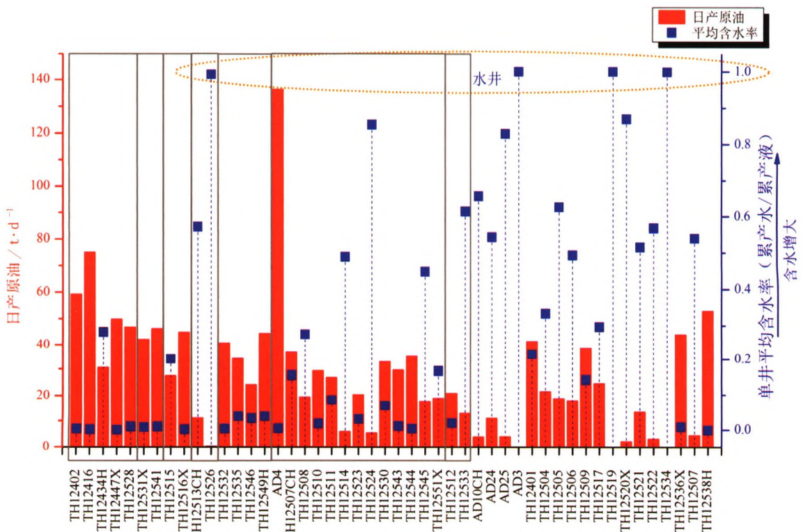
图 2 研究区生产井的日均原油产量和平均含水率
