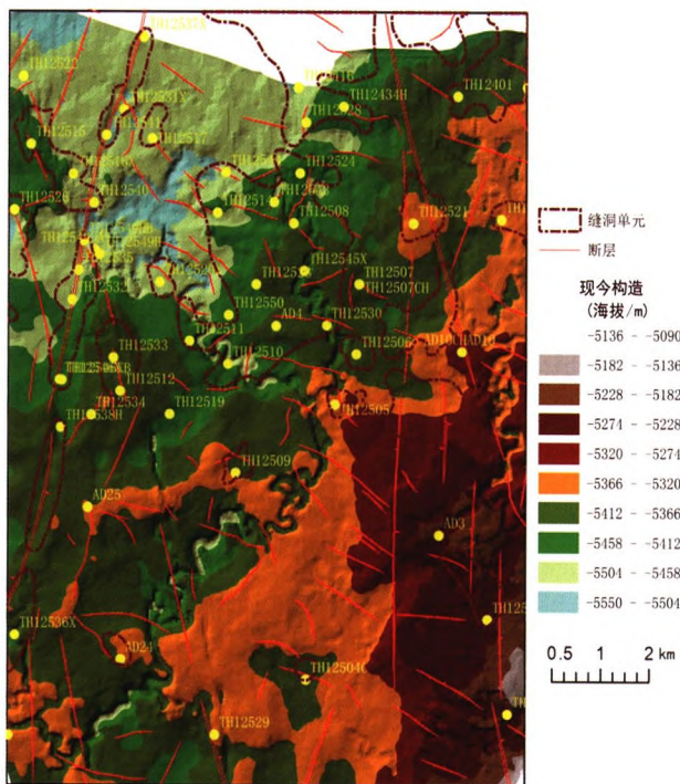
图 7 T_7^0 地震波反射界面的现今构造
