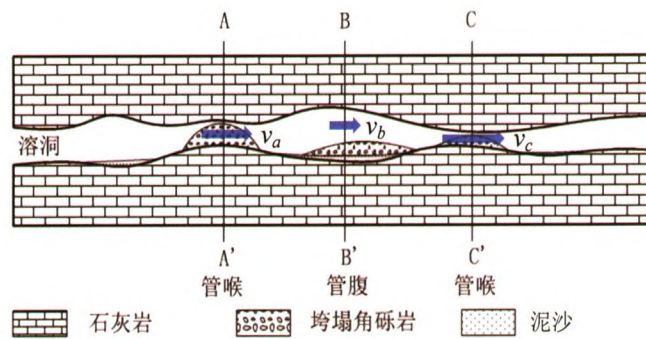
图12 化学充填作用所致渗透屏障的形成模式
