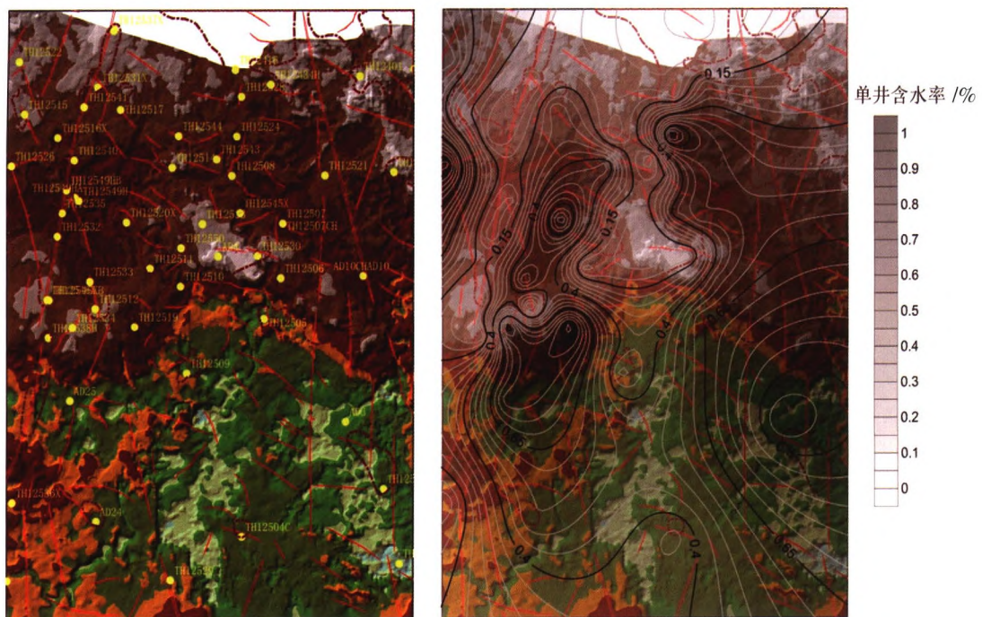
图9 海西晚期热液活动期的 T_7^0 界面与现今生产井的含水等级等值线对比
