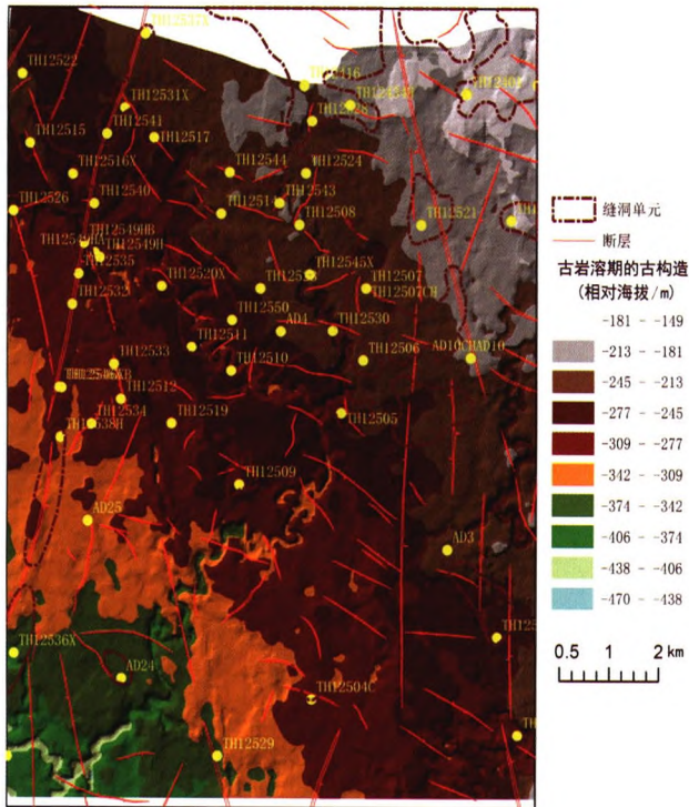
图 6 T_7^0 地震波反射界面的古构造
