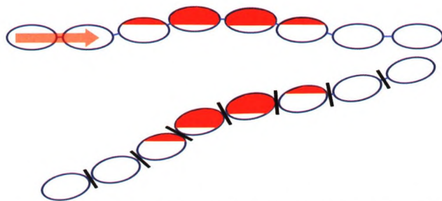
图13 研究区的油水关系发展模式(红色代表石油,黑色粗短线代表渗流屏障)
