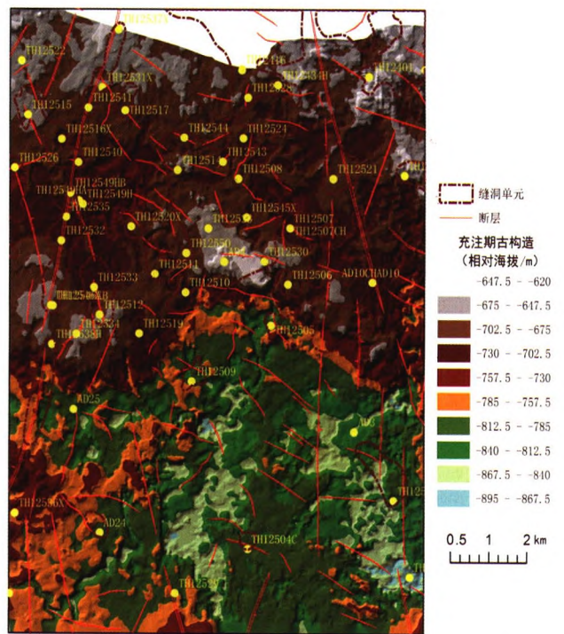
图 8 T_7^0 地震波反射界面在海西晚期的古构造
