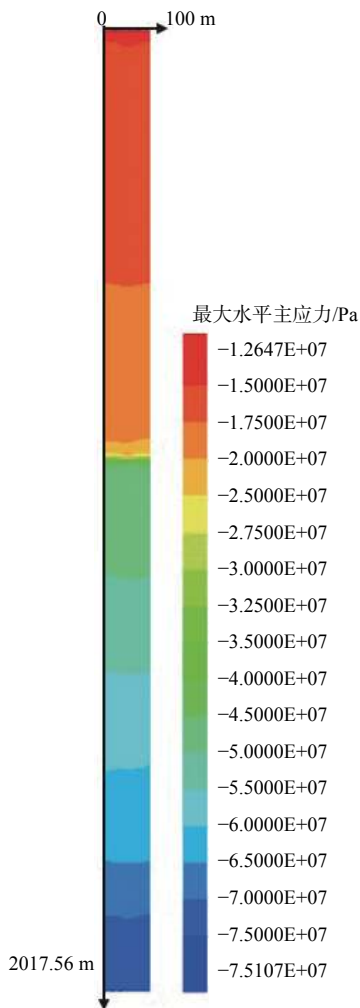
图 8 最大水平主应力云图 Fig. 8 Cloud of maximum horizontal principal stress
