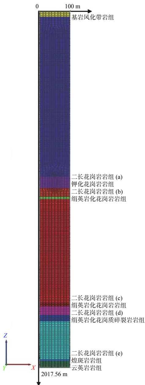
图 7 地质模型图和网格细节图 Fig. 7 Geological model map and grid details
