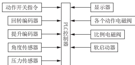
图 6 电气控制系统框图
