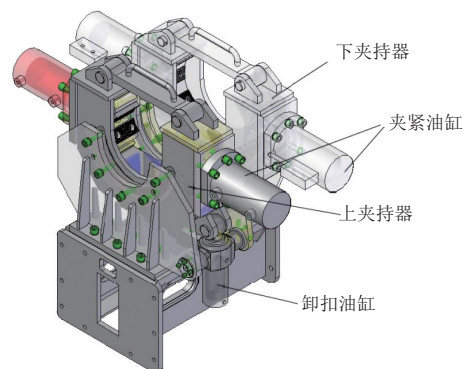
图 4 夹持器结构示意图
