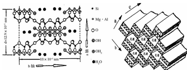
图 1 凹凸棒石晶体结构示意图 [5]
