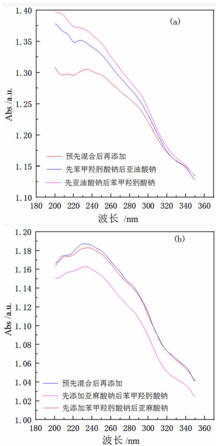
(a) 苯甲羟肟酸钠 + 亚油酸钠体系; (b) 苯甲羟肟酸钠 + 亚麻酸钠体系
