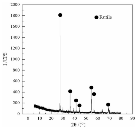
图 1 试验样品 XRD 图 Fig. 1 XRD analysis of experimental sample
