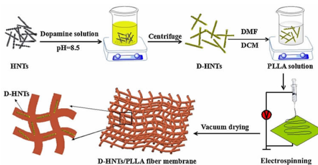
图7 静电纺丝制备 D-HNTs/PLLA 复合纤维流程
