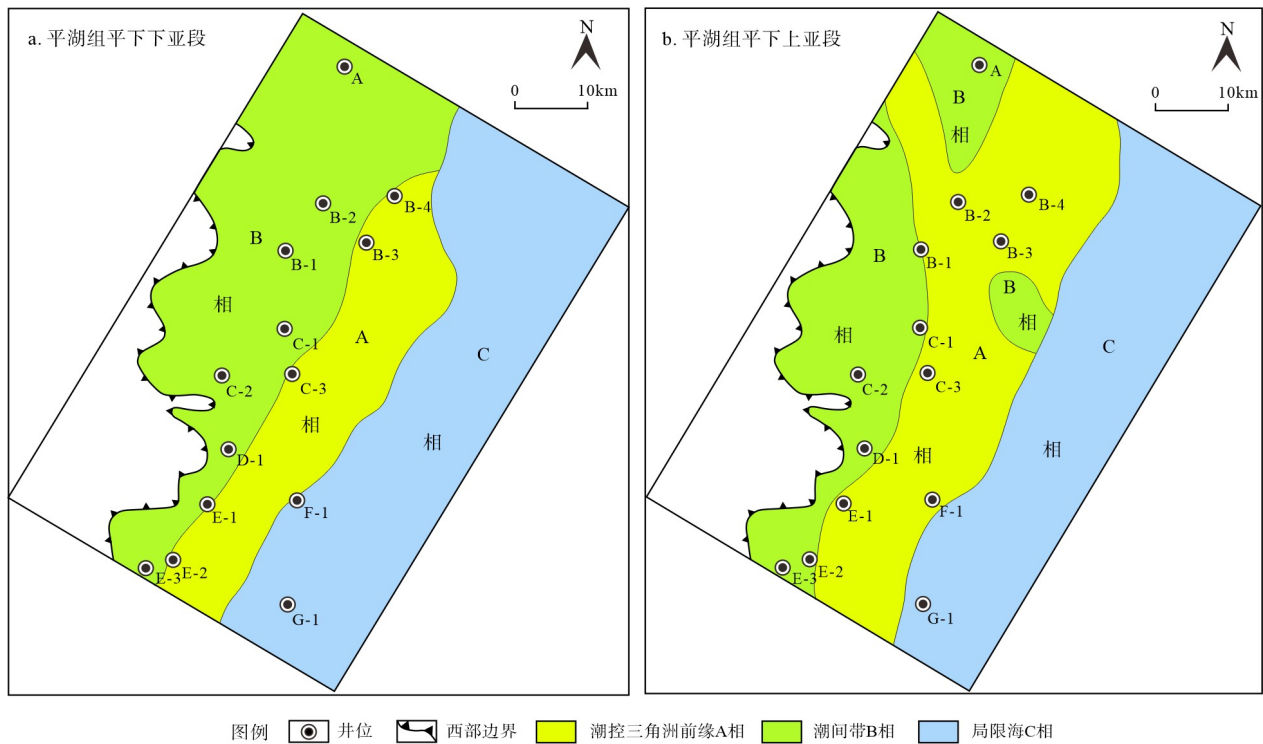
图6 西湖凹陷平北地区平湖组下段烃源岩有机相平面分布图
