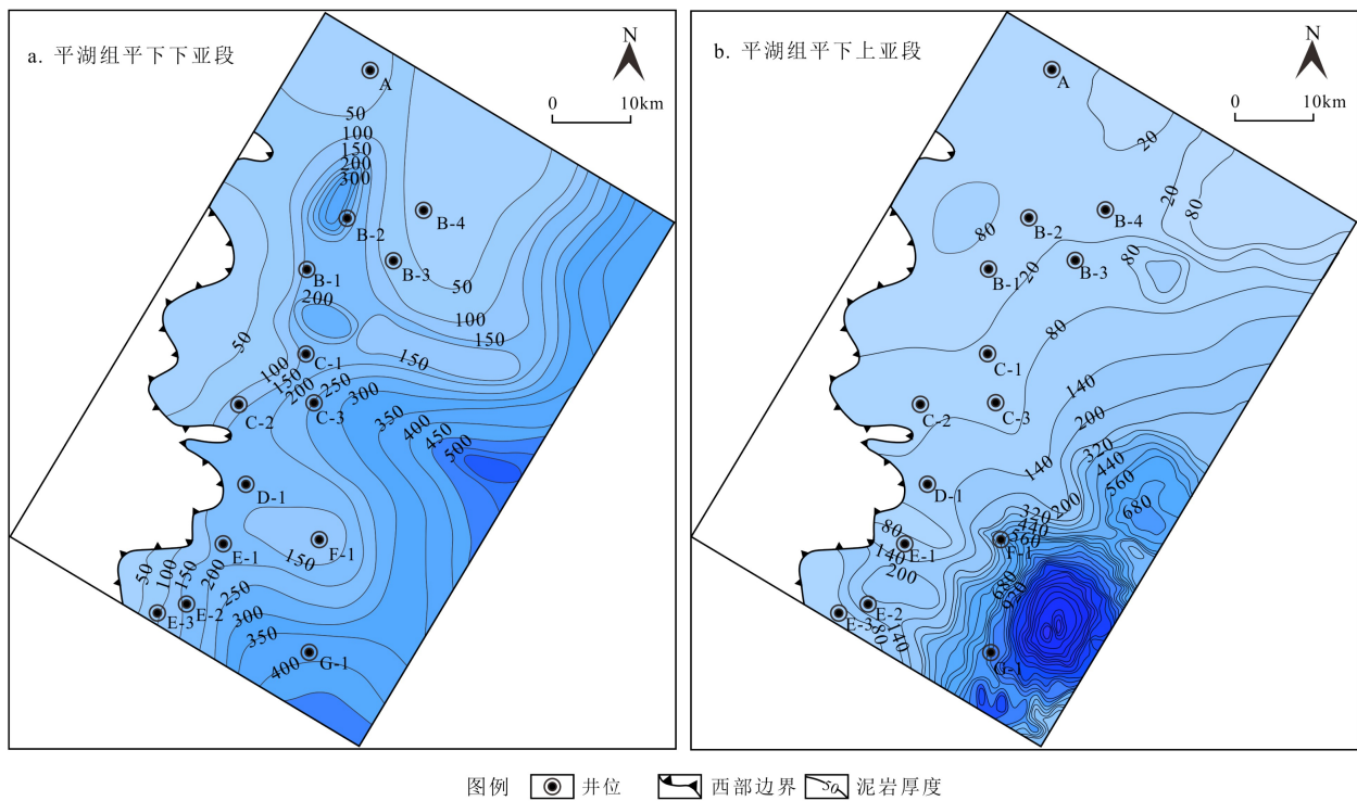
图8 西湖凹陷平北地区平湖组下段泥岩厚度平面分布图
