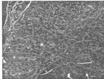
下表皮(×200)
