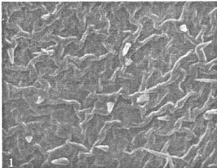
上表皮(×200)
