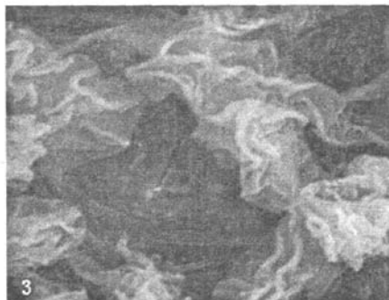
气孔(×1400)
