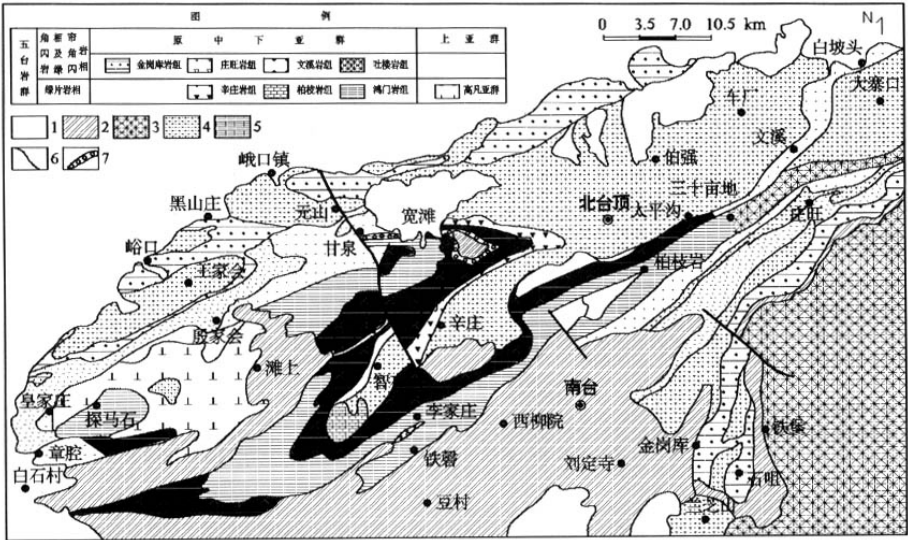
图 1 五台山地质略图
