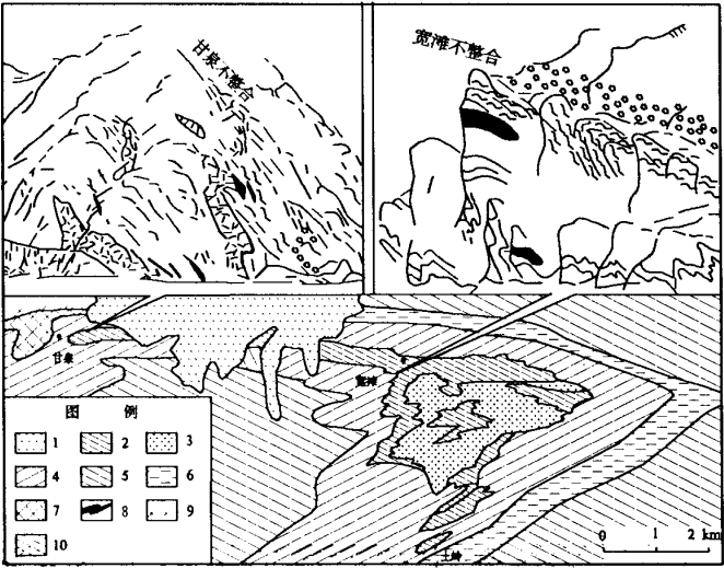
图 2 甘泉、宽滩不整合露头素描与区域地质略图
