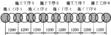
图 1 CMW 工法施工顺序图
