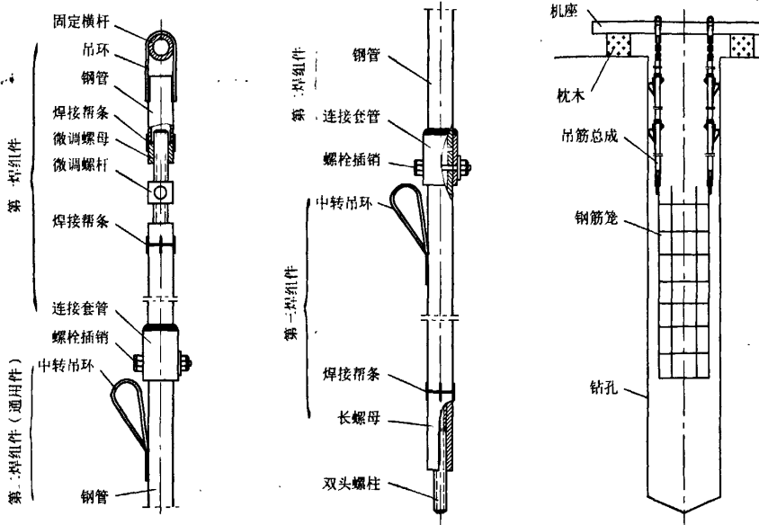
图1 螺栓连接可拆卸吊筋详图和安装示意图
