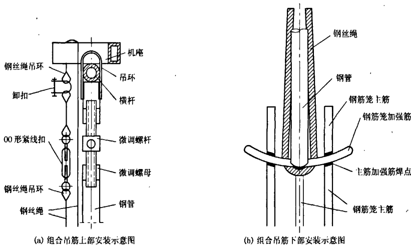
图2 钢丝绳加套管可拆卸组合吊筋安装示意图
