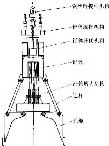
图1 CZ-2000型冲抓锥结构示意图
