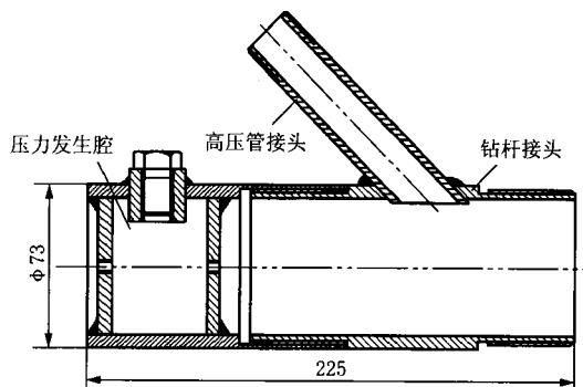
图 3 自行设计制造的液压发生器
