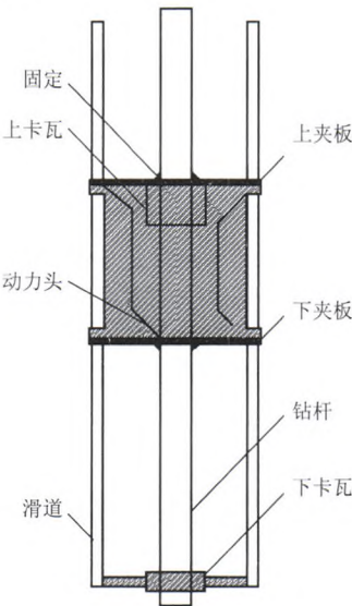
图 1 U8 型钻机夹板示意图
