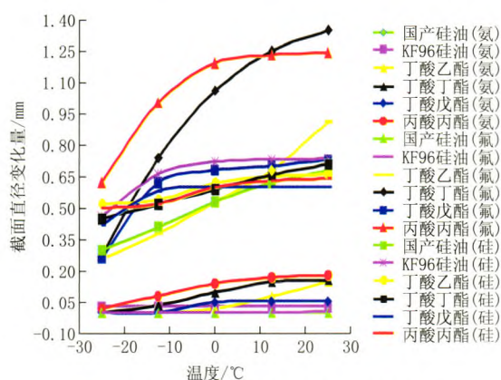
图5 截面直径变化量随温度变化的曲线
