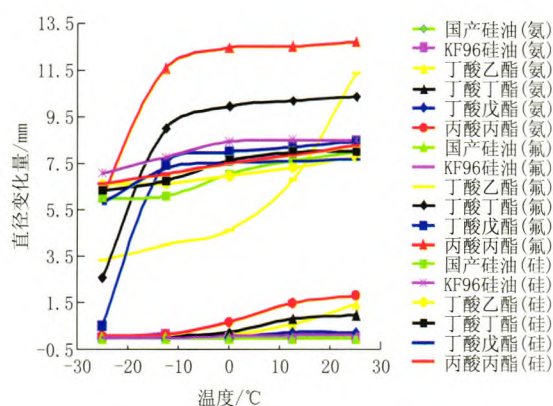
图4 直径变化量随温度变化的曲线
