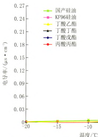
图 1 350 mL 介质中加入 16 \text{ cm}^3 冰屑的电导率随温度变化曲线
