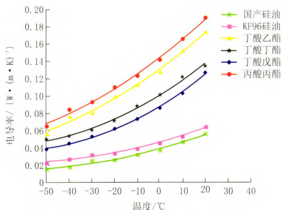
图 3 6 种介质的导热系数随温度变化的曲线
