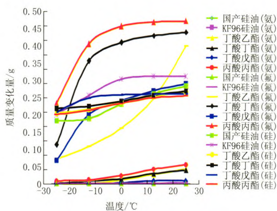
图6 质量变化量随温度变化的曲线
