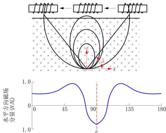
图 7 水平方向磁场分量及其分布
