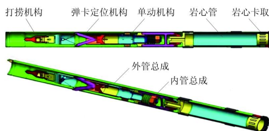
图3 大直径绳索取心钻具结构
