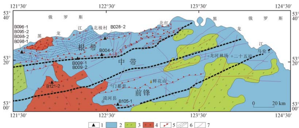
1—采样地点; 2—中—晚侏罗世额尔古纳河群; 3—晚侏罗世—早白垩世火山岩; 4—前寒武纪花岗岩; 5—逆冲断裂; 6—糜棱岩带; 7—断层
