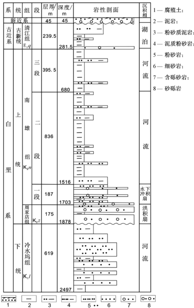
图4 白垩—古近系地层序列特征 [11]
