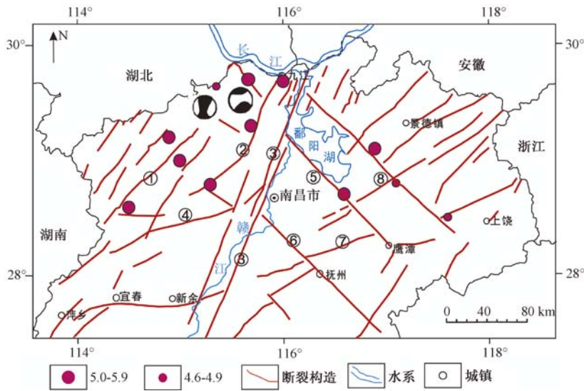
①武宁—铜鼓断裂；②九江—靖安断裂；③湖口—吉安断裂（赣江断裂）；④宜丰—新建断裂； ⑤余干—鹰潭断裂；⑥抚河断裂；⑦宜春—东乡断裂；⑧余干—婺源断裂
