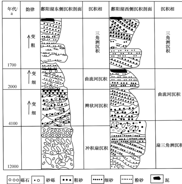
图7 鄱阳湖东西两侧沉积垂向特征 [45,47]
