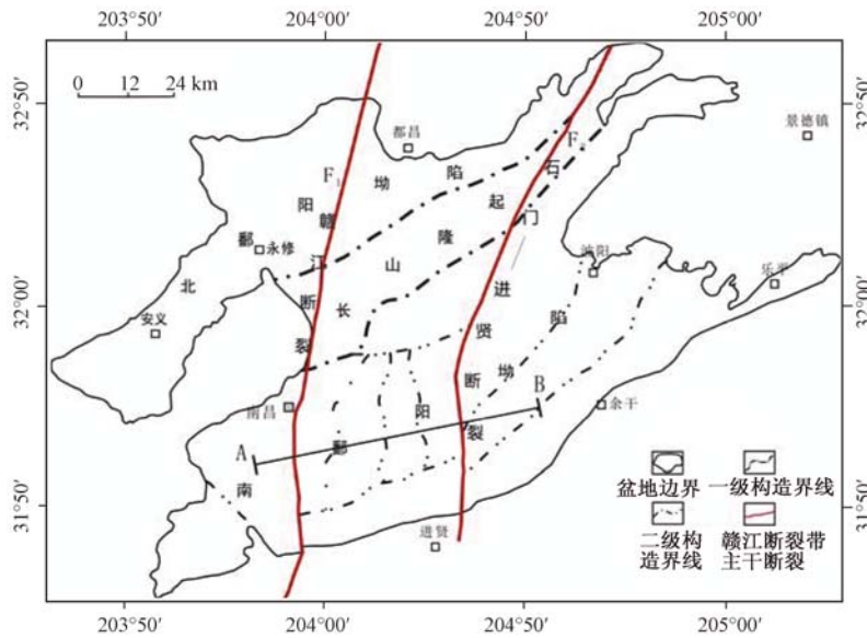
图2 鄱阳湖盆地构造分区简图 (据周松源等 [22] )
