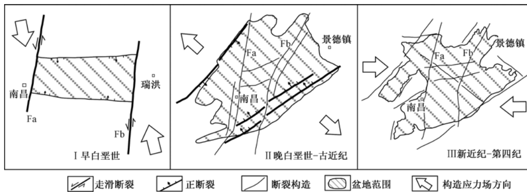
I—早白垩世拉分盆地雏形出现；II—晚白垩—古近纪盆地稳定扩张阶段；III—新近纪—第四纪盆地萎缩，呈整体拗陷阶段，受多条断裂影响；Fa—赣江断裂；Fb—进贤—石门街断裂
