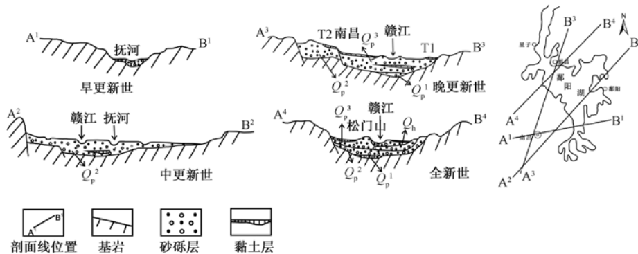
图6 第四纪各时期鄱阳湖盆地剖面图 [33]
