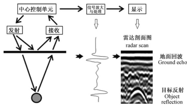
图 1 地质雷达工作原理示意图
