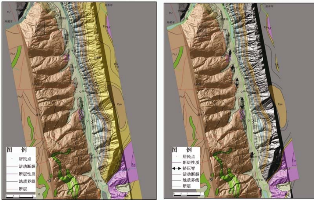
图6 小江断裂形成的地貌特征
