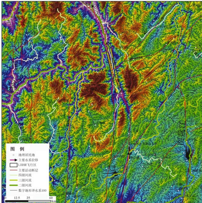
图7 东川周边小江断裂主要的错断裂水系
