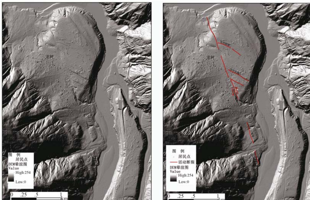
图5 龙树阶地被小江断裂切割的地貌特征
