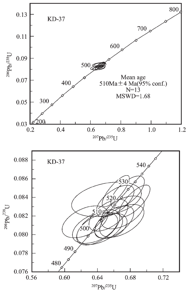
图4 库地蛇绿岩中石英辉长岩 (KD37) 的锆石 SHRIMP-II 测年
