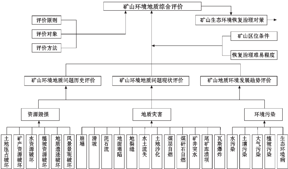
图1 矿山环境地质问题综合评价体系流程
