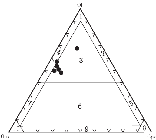
图5 超基性岩标准分子Ol-Opx-Cpx分类图解
