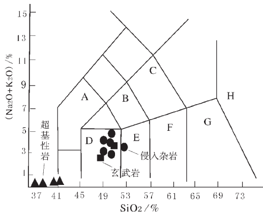
图4 苏巴什蛇绿混杂岩TAS图解
