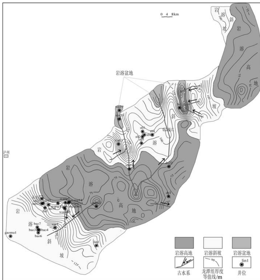
图6 川东南地区茅口组岩溶古地貌单元划分
