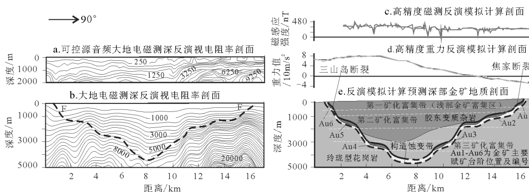
图4 地球物理反演模拟深部金矿地质剖面
