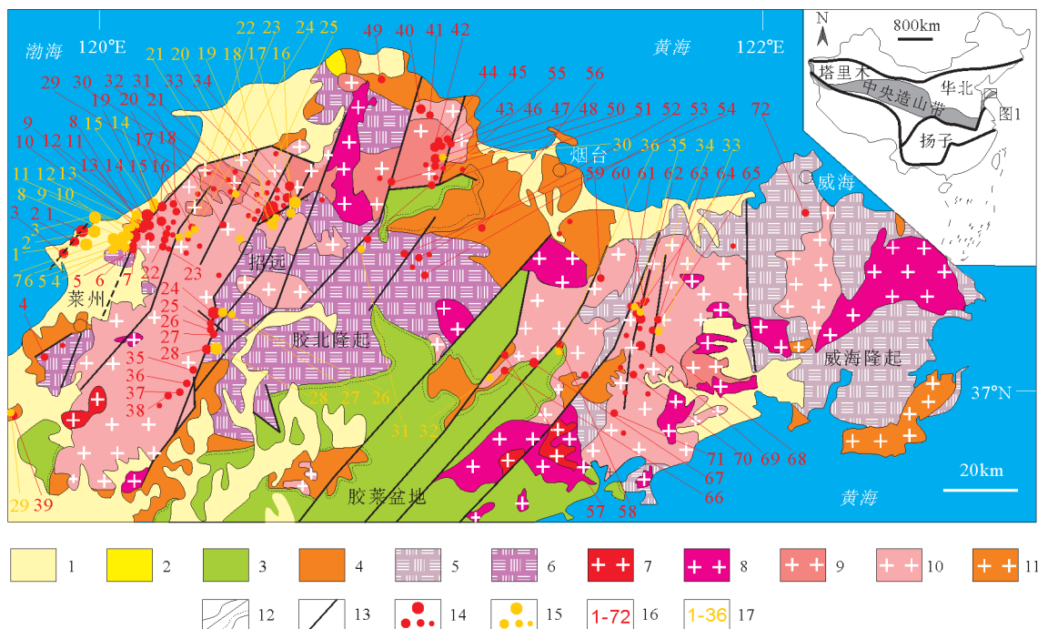
图1 胶东地区区域地质及金矿床分布
