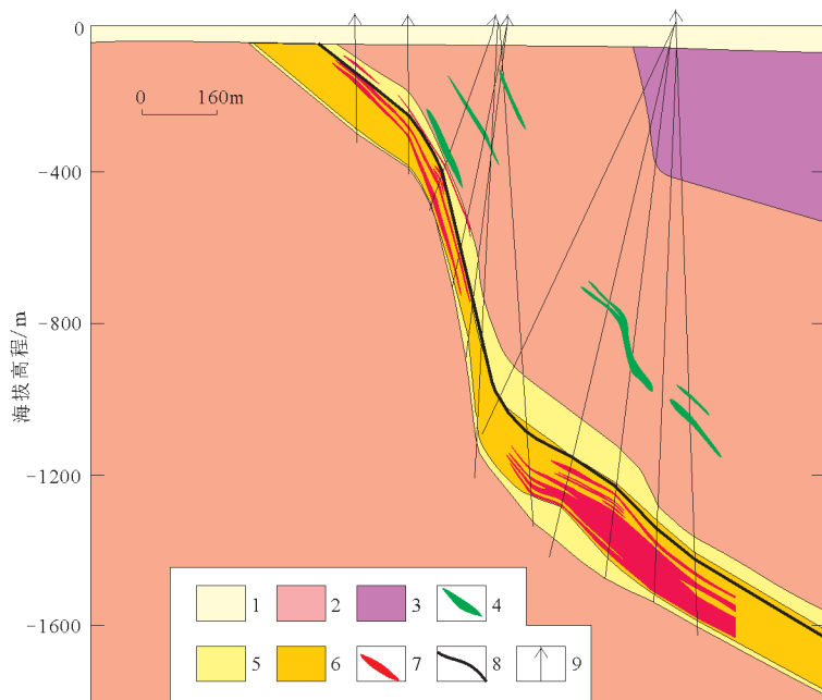
图2 三山岛北部海域矿区第30勘探线地质剖面
