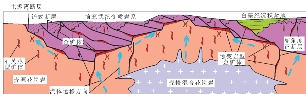
图3 胶东金矿热隆-伸展成矿理论模型剖面示意图
