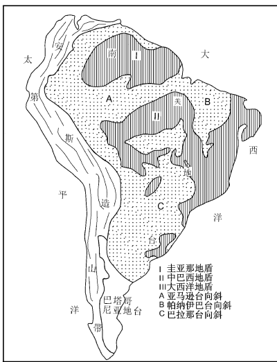
图 1 南美地台地质构造分区略图 [1]
