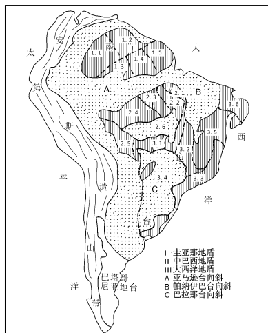
图 4 南美地台 III 级成矿亚带划分示意图
