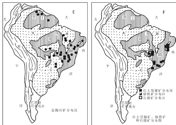
图 3 南美地台金刚石矿和红土型镍矿分布图(图例同图 1)
