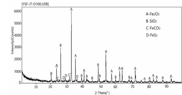
图 1 原矿 XRD 分析图 Fig. 1 XRD pattern of raw ores
