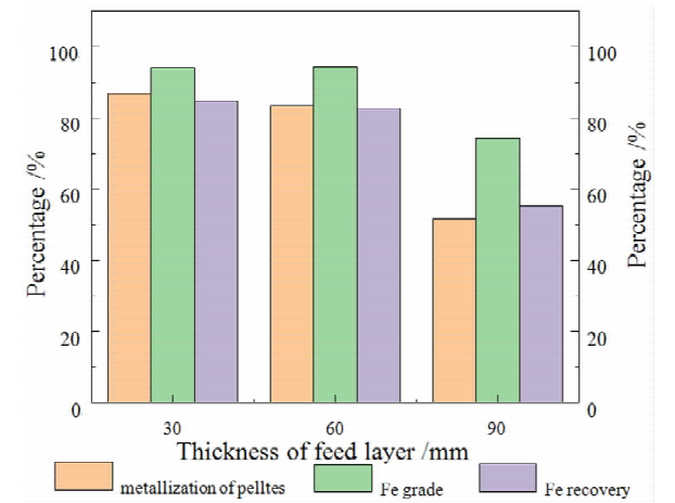
图 6 料层厚度对指标的影响 Fig. 6 Influence of thickness on reduction parameters
