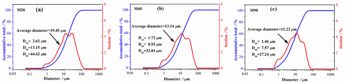
图2 天然辉钼矿尺寸分布图 (a) M30、(b) M60 和 (c) M90
