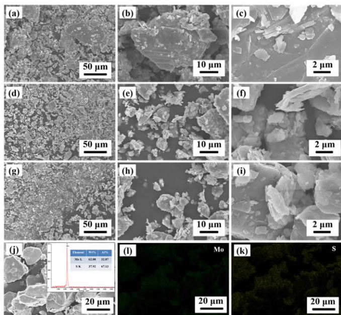
图 4 天然辉钼矿 SEM 图谱(a - c) M30、(d - f) M60、(g - i) M90 和(j - l) 辉钼矿的 EDX 元素映射图 Fig. 4 SEM spectra of natural molybdenite at (a - c) M30, (d - f) M60, (g - i) M90, and (j - l) EDX elemental mapping images of molybdenite
