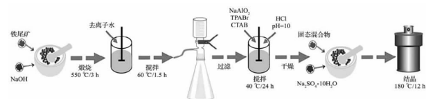
图1 铁尾矿制备介孔微球工艺流程 [116]
