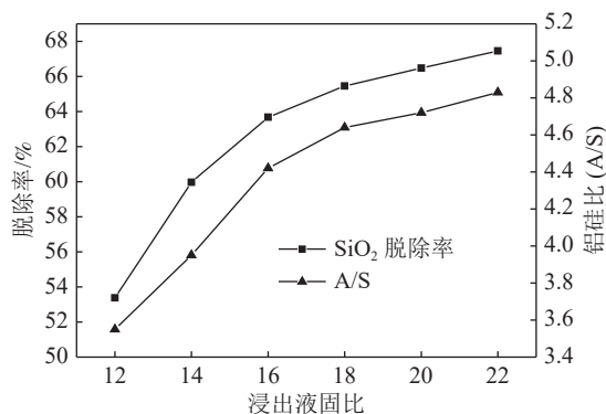
图6 浸出液固比对脱硅的影响
