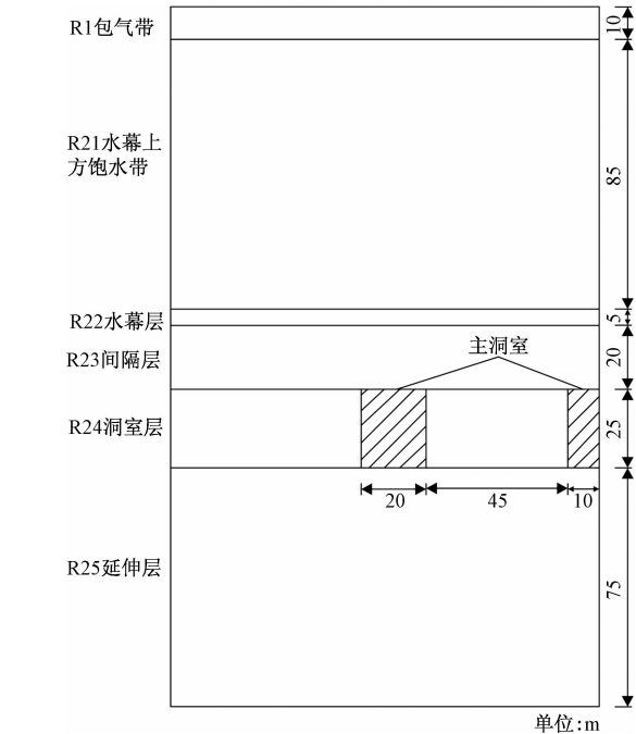
图 2 丙烷洞库概化剖面 Fig.2 Propane cavern section for parameter generalization
