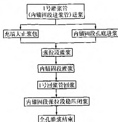
图2 灌浆工艺流程图
