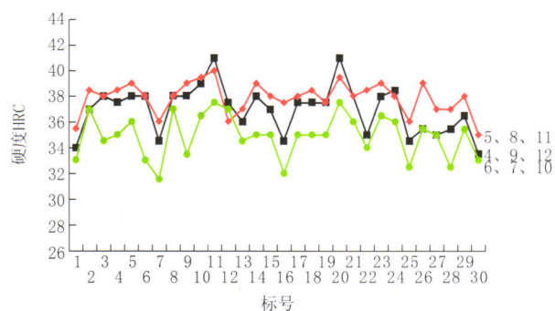
图14 第4次磨1 mm后硬度曲线
