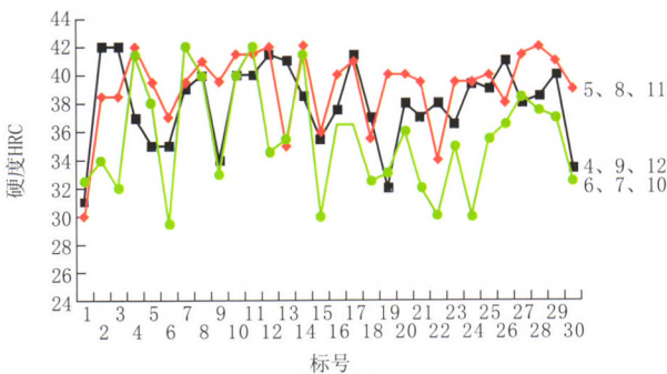
图 10 胎体唇面表面硬度曲线
