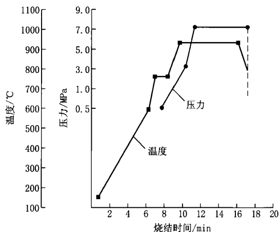
图6 试验用金刚石钻头烧结工艺曲线
