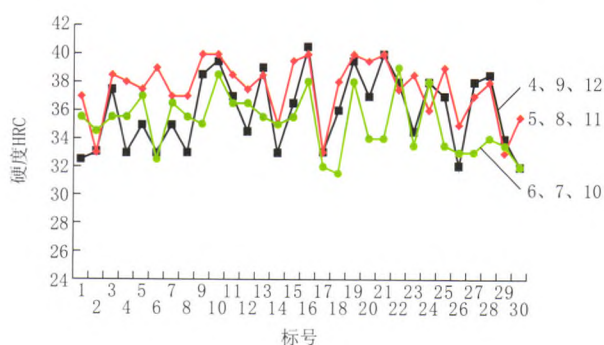
图16 第6次磨1 mm后水口附近硬度曲线
