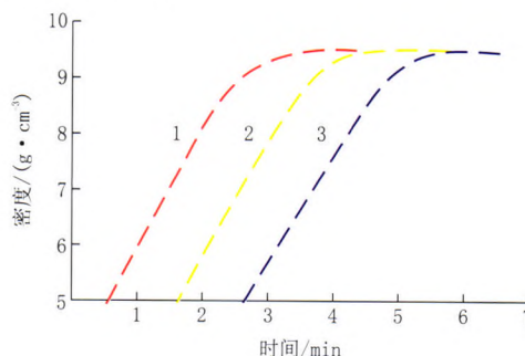
图4 胎体密度与时间的关系
