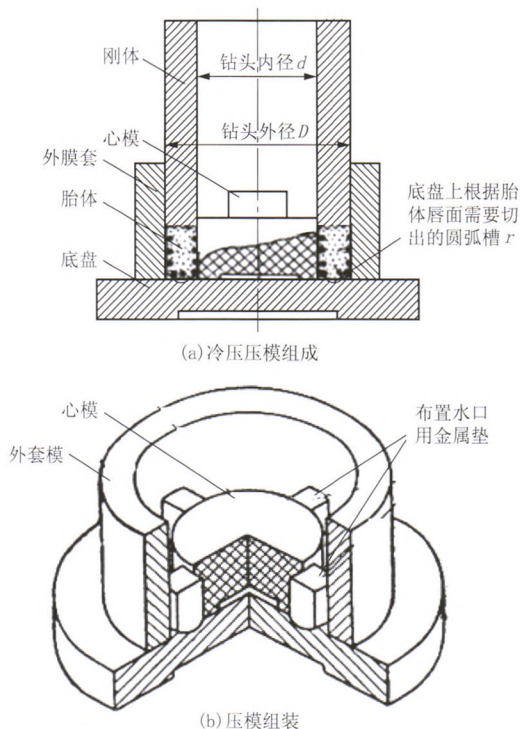
图8 俄罗斯使用的冷压烧结模具
