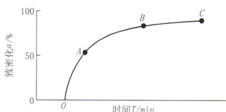
图3 致密化过程与时间的关系
