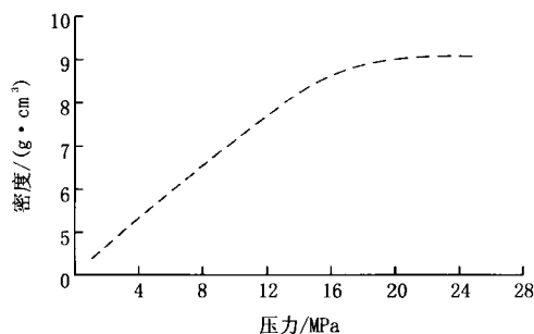
图5 胎体密度与热压压力的关系
