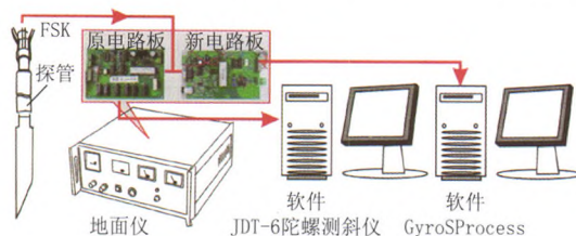
图 8 软件 J6 与 GyroSPProcess 对比试验模型
