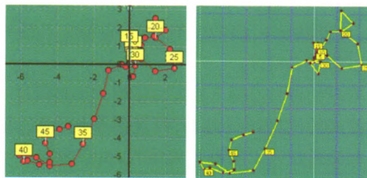
图 9 J6 (左) 与 GyroSPProcess (右) 软件所获得同一钻孔的轨迹
