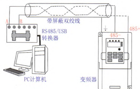
图 4 PC 计算机、转换器、变频器组成的 ModBus 网络
