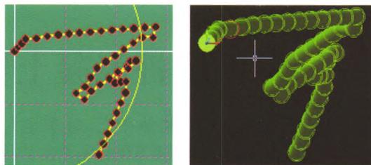
图 7 在 GyroSPProcess (左) 和 AutoCAD (右) 中的钻孔轨迹
