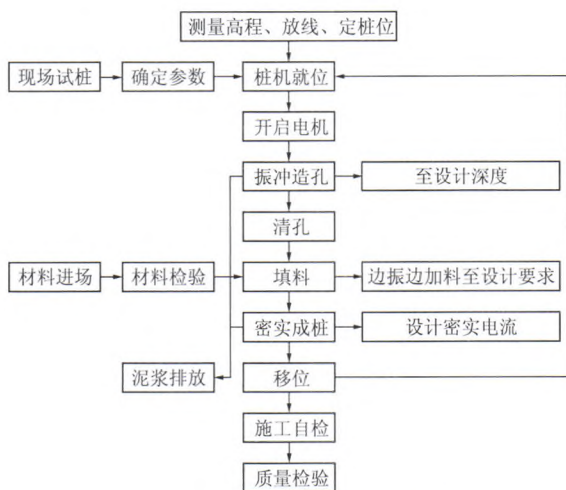
图 1 振冲碎石桩施工工艺流程图
