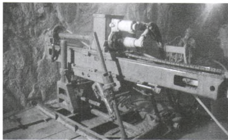
图7 洞库现场水平水幕孔钻孔
