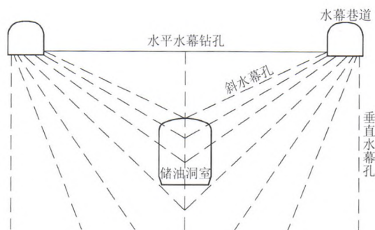
图2 人工水幕示意图
