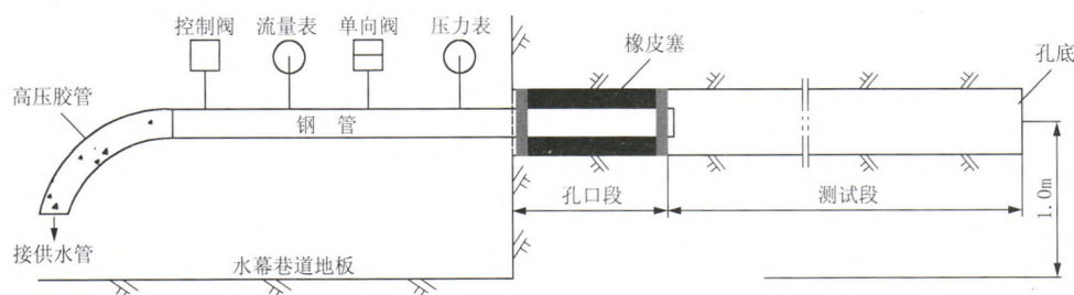
图5 水幕孔孔口装置
