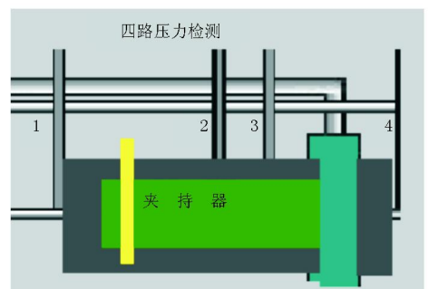
图 2 岩心四路压力检测示意图
