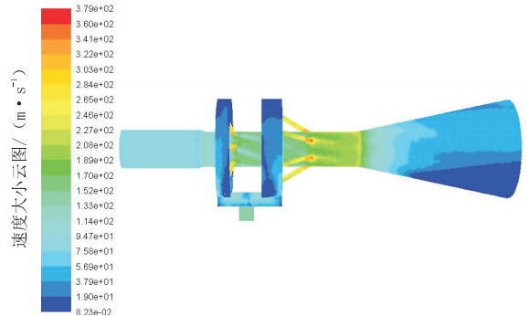
图6 消泡器内部速度场立体云图
