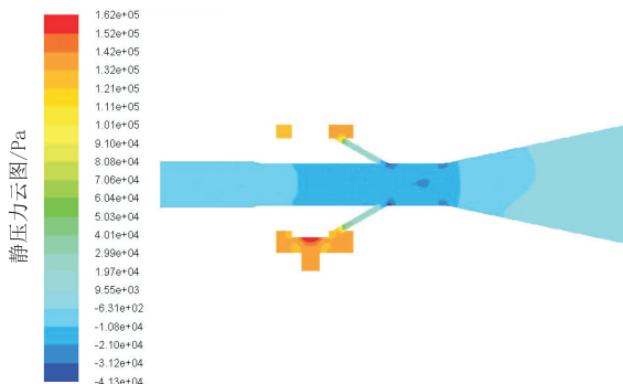
图 10 消泡器内部压力剖面云图
