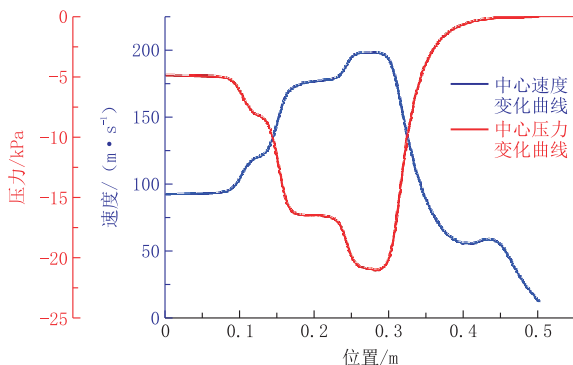
图 11 中心速度、压力变化对比曲线图
