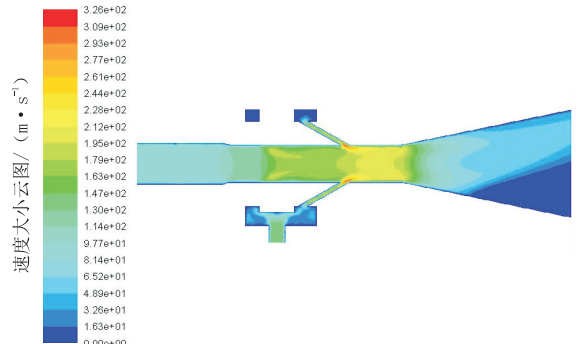
图7 消泡器内部速度场剖面云图
